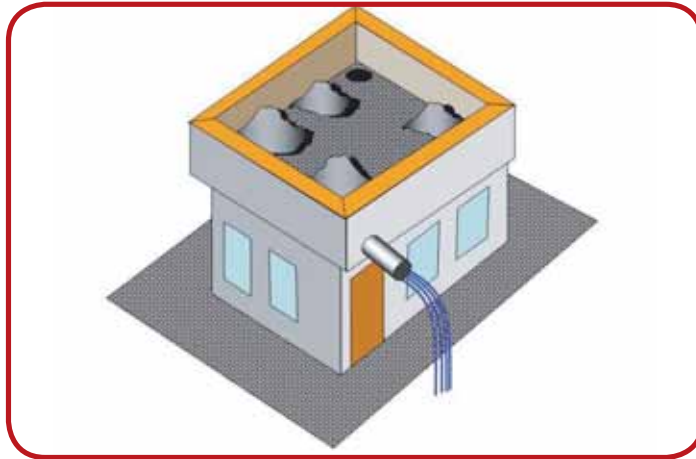
Figura 53. La acumulación de cenizas en los techos debe retirarse antes de producir el colapso del tejado. Hay que evitar que obstruya los sistemas de desagüe, por lo que deben cerrarse e instalarse canalones auxiliares.
