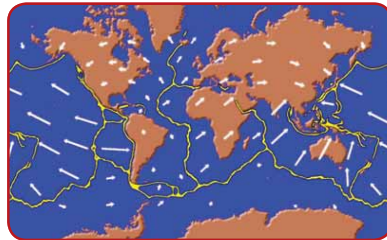
Figura 2. Principales placas tectónicas y dirección de movimiento.
