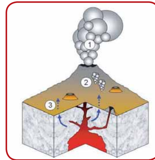
Figura 25. 1 penacho de gases, 2 fumarolas, 3 difusión de gases
