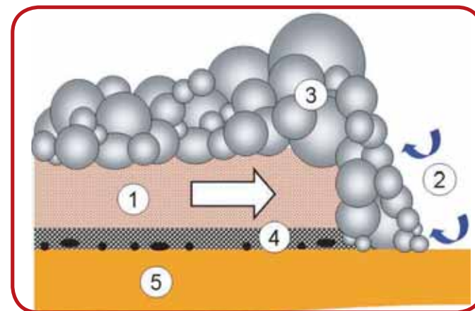
Figura 27. Anatomía de una colada piroclástica: 1 masa de gases y cenizas a alta temperatura, 2 incorporación de aire, 3 nube acompañante formada por gases y partículas muy finas que se escapan del flujo, 4 nivel de base donde se van depositando los bloques más pesados, 5 superficie sobre la que se desplaza.
