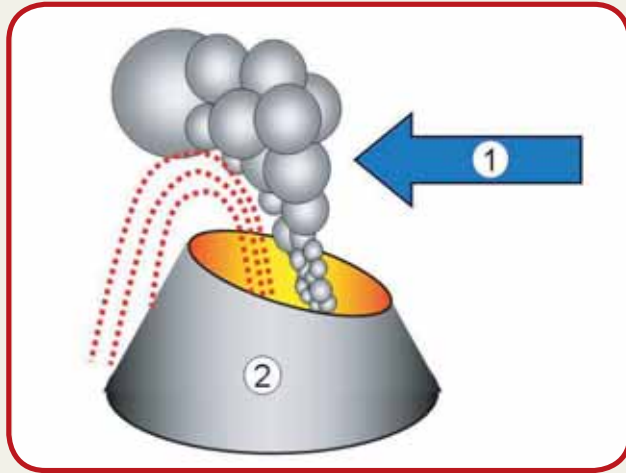
Figura 32. Cuando hay un viento fuerte (1), el cono (2) crece asimétrico, ya que las escorias son arrastradas por el viento.
