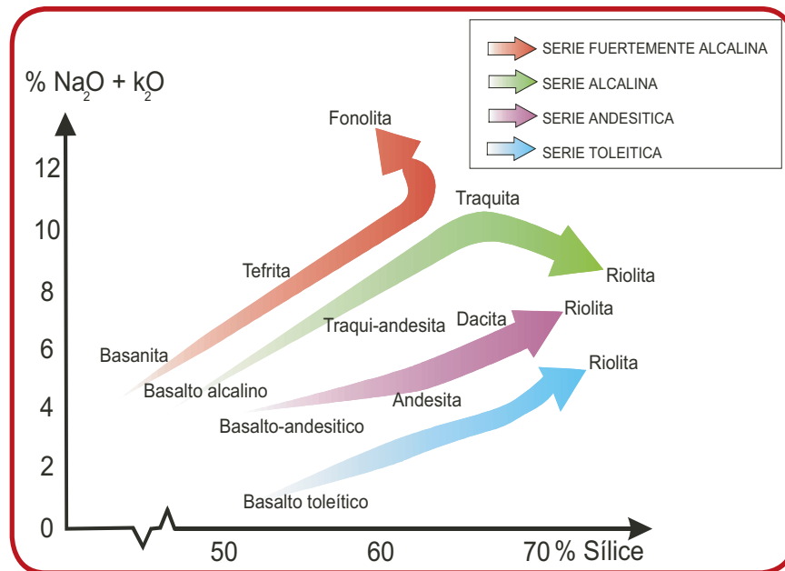
Figura 8. Tipo de rocas en función del porcentaje de Sílice y Alcalis.
