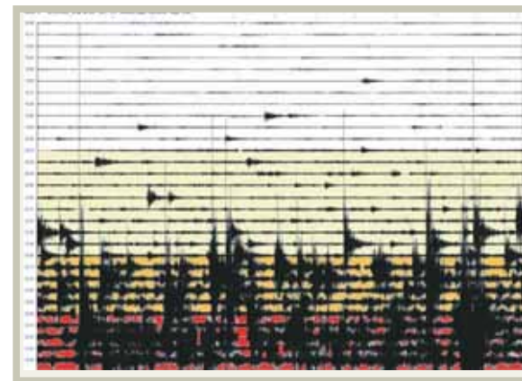
Incremento de actividad sísmica en el volcán Etna al inicio de la erupción de 2002. INGV Italia.
