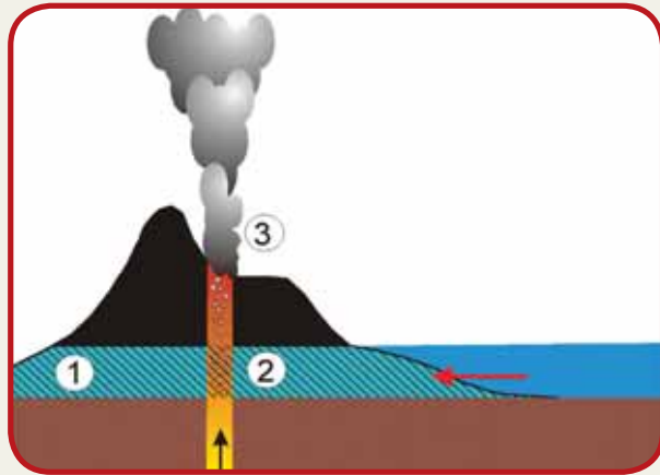
Figura 13. 1 Nivel freático; 2 incorporación de agua al magma; 3 incremento de la explosividad por el aumento de los gases.
